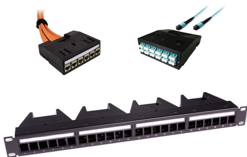
NGC1710
